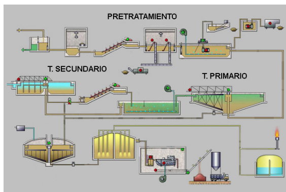
Esquema simple de una Estación Depuradora de Aguas Residuales.
