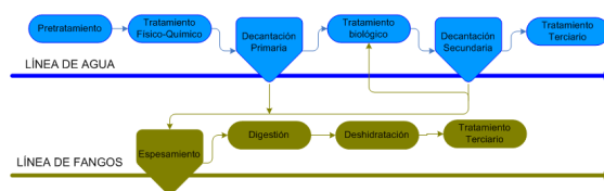
Esquema simple de una EDAR
