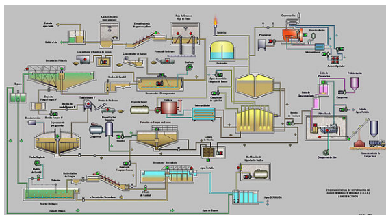
Esquema detallado de una Estación Depuradora de Aguas Residuales.
